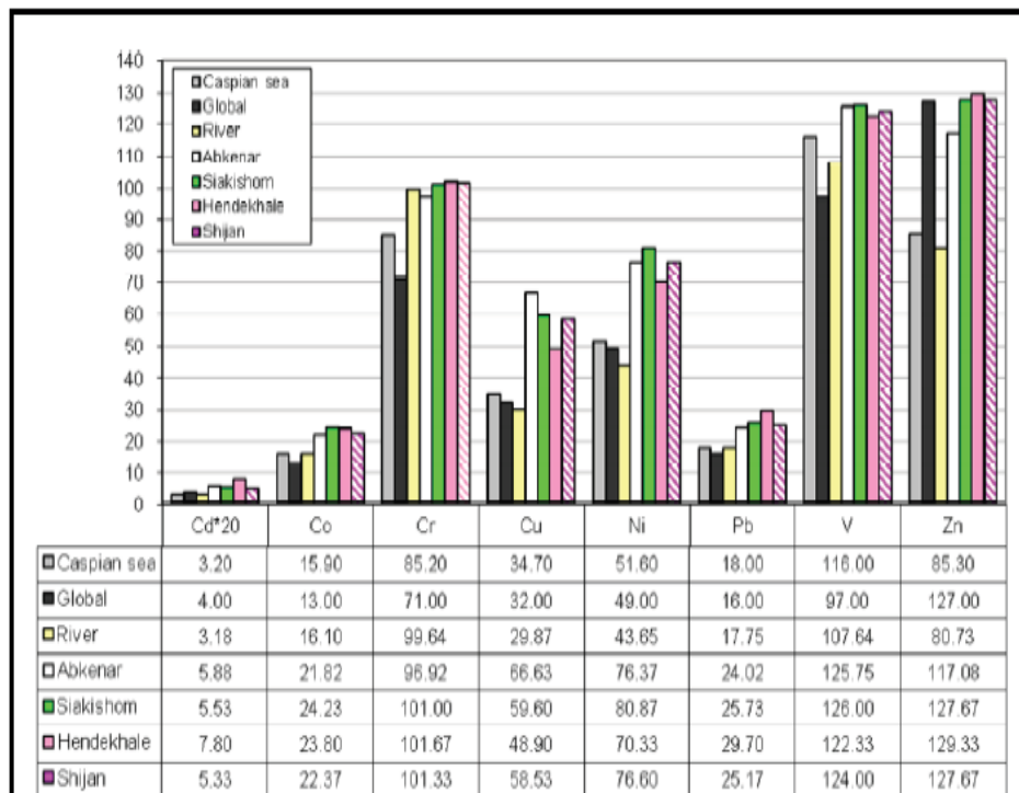
شکل ۷- مقایسه میانگین غلظت عناصر سنگین در استانداردهای رودخانه ای و دریایی با بخش های چهارگانه تالاب انزلی
