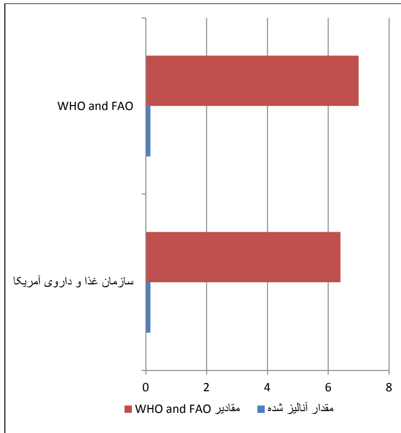
شکل ۶- مقایسه میانگین غلظت کادمیم در بافت نرم صدف با مقادیر سازمان غذا و داروی آمریکا و WHO and FAO
