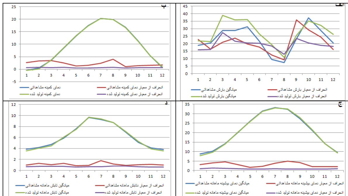
شکل ۲- مقایسه مقادیر دیده بانی و مدل شده برای متغیرهای الف. بارش، ب. دمای کمینه، ج. دمای بیشینه و د. تابش ایستگاه سینوپتیک پارس آباد برای دوره ۲۰۰۹-۱۹۹۹
