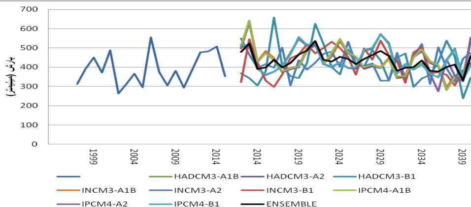
شکل ۵- مقایسه بارش دوره آماری با بارش مدل های GCM و سناریوهای انتشار در ایستگاه مشکین شهر
